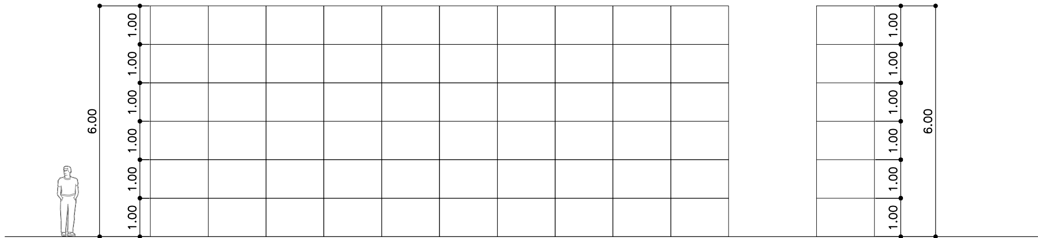
ELEVAÇÕES FRONTAL E LATERAL ESQUEMÁTICAS DOS ANDAIMES LOCAL: COBERTURA PRINCIPAL ESC.: 1:100 EM METROS
