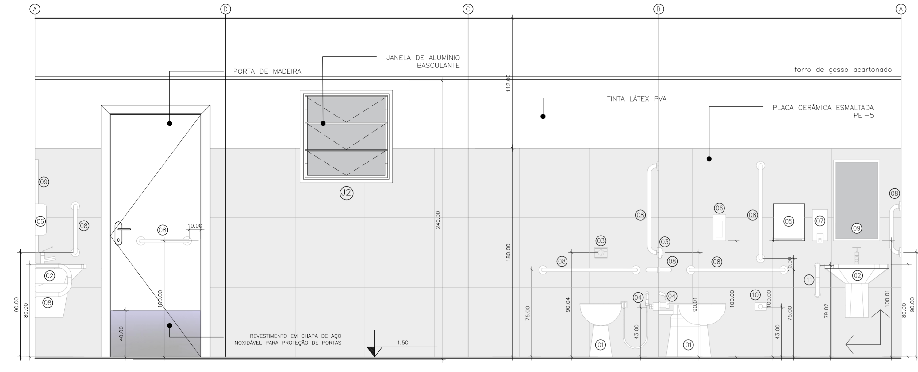
AMPLIAÇÃO - W.C. PCD ESCALA 1:20
