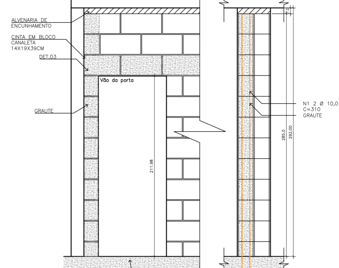
ELEVÇÃO PROJETO ESTRUTURAL - W.C. PCD ESCALA 1:20
