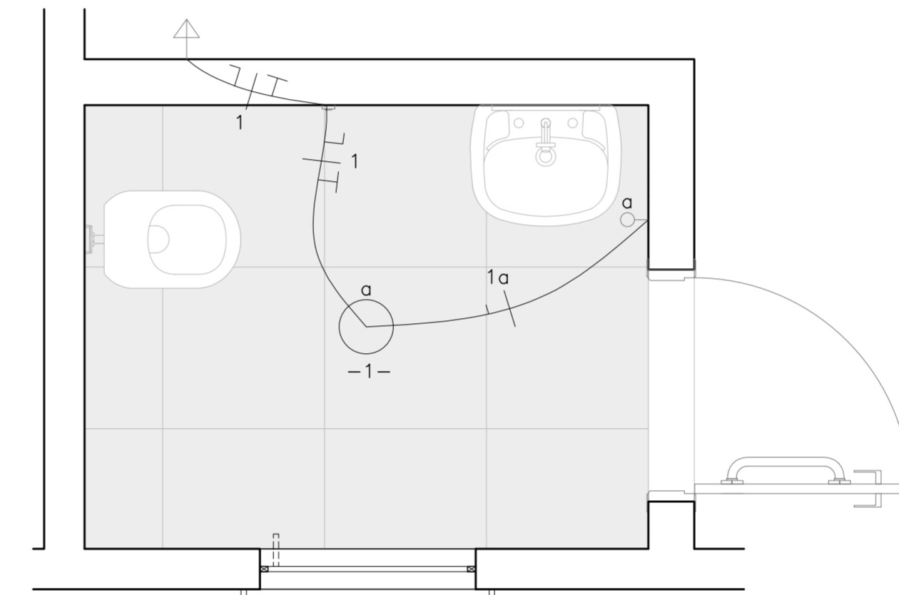
INSTALAÇÃO ELÉTRICA - W.C. PCD ESCALA 1:20
