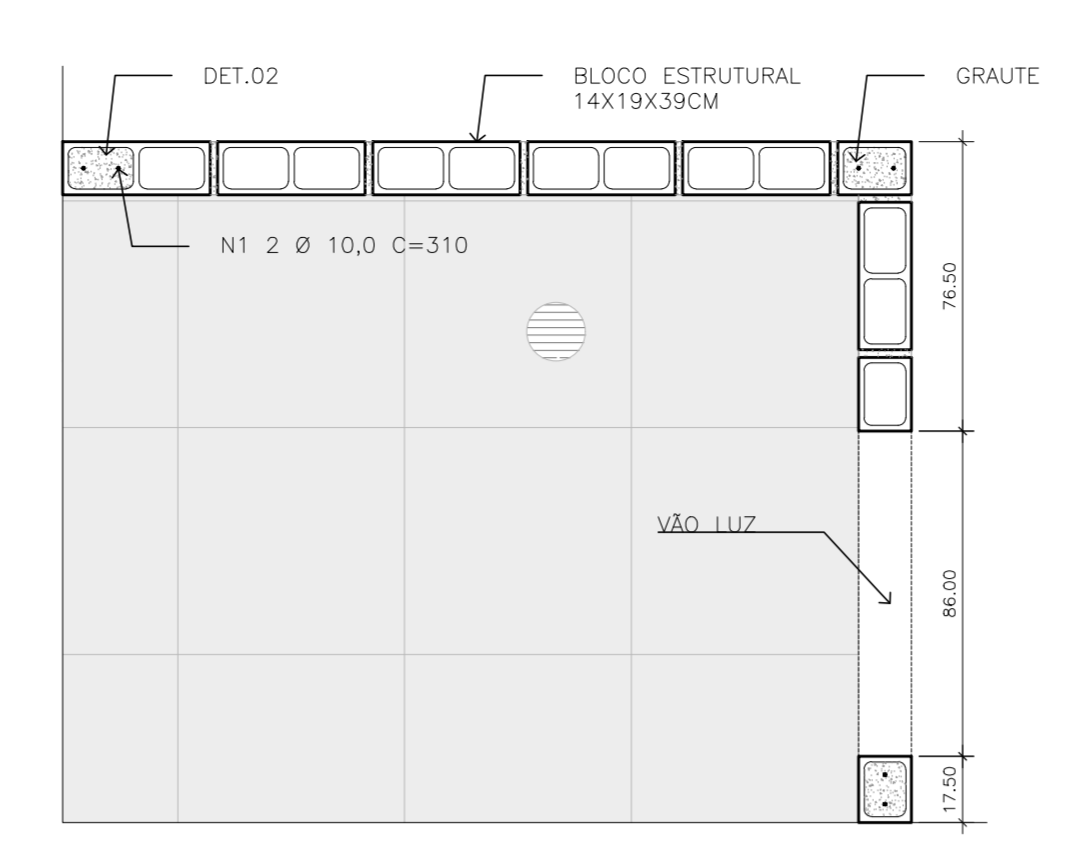
PLANTA PROJETO ESTRUTURAL - W.C. PCD PAREDE ESTRUTURAL ESCALA 1:20
