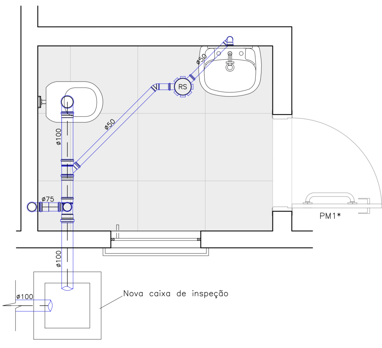
INSTALAÇÃO DE ESGOTO SANITÁRIO - W.C. PCD
