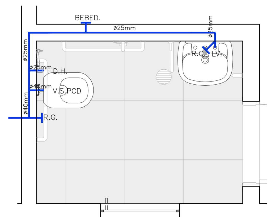
INSTALAÇÃO DE REDE DE ÁGUA FRIA - W.C. PCD ESCALA 1:20
