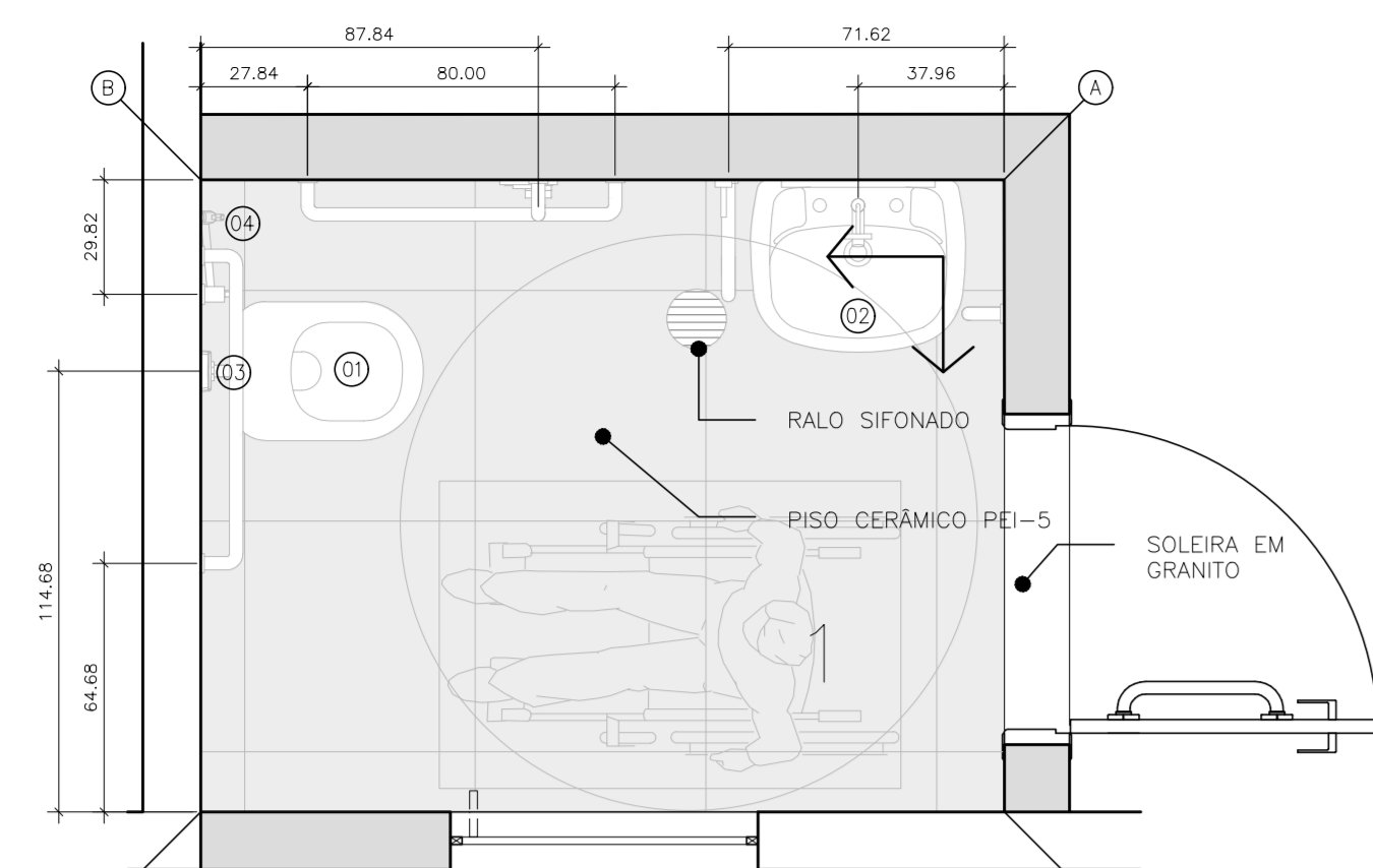
LAYOUT - W.C. PCD ESCALA 1:20
