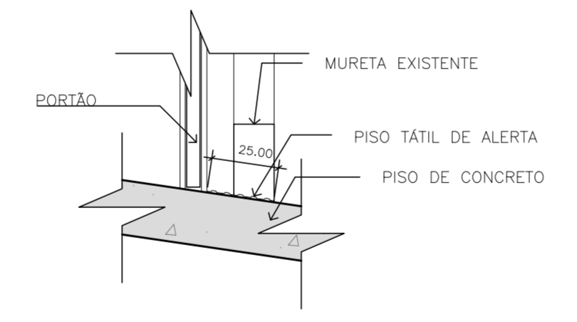
CORTE PISO TÁTIL DE ALERTA - ACESSO PRINCIPAL ESCALA 1:20
