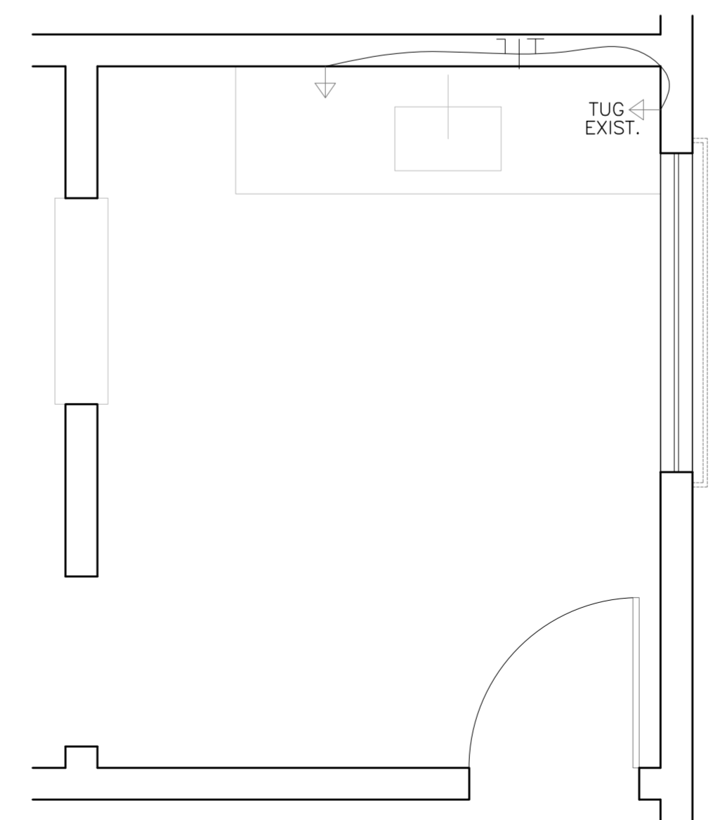
INSTALAÇÃO ELÉTRICA - COZINHA ESCALA 1:25
