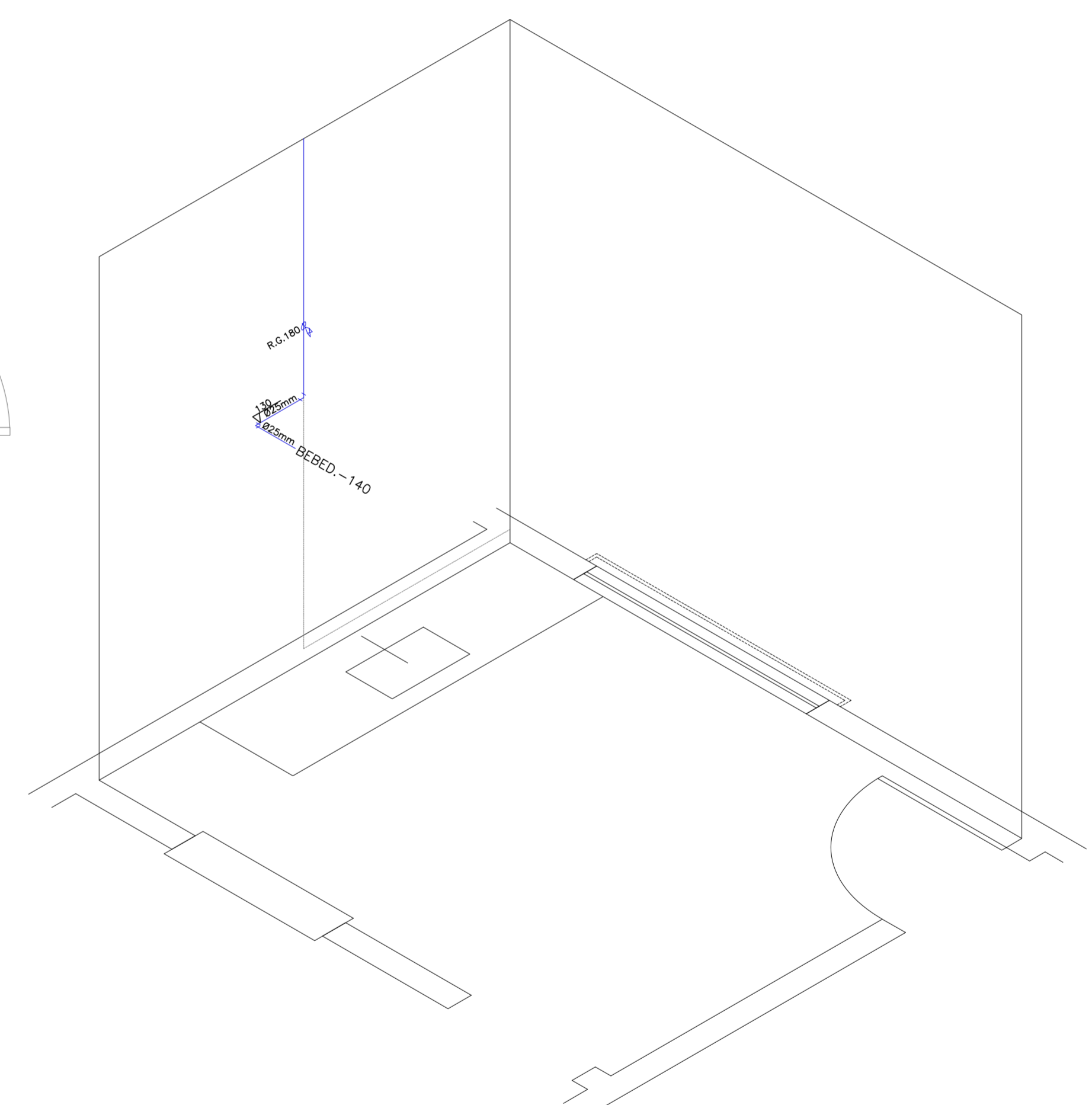
ISOMÉTRICA ÁGUA FRIA - COZINHA ESCALA 1:25
