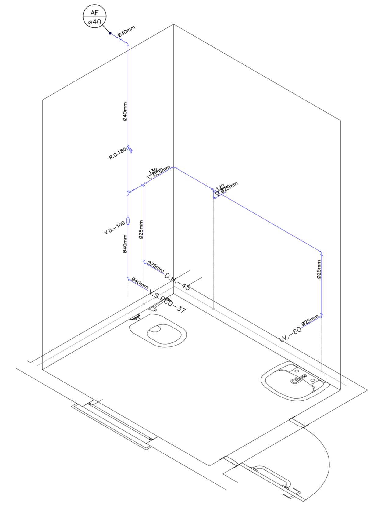
ISOMÉTRICA ÁGUA FRIA - W.C. PCD ESCALA 1:25
