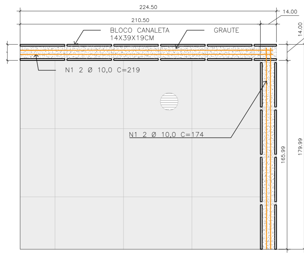
PROJETO ESTRUTURAL - W.C. PCD VIGAS BALDRAMES ESCALA 1:20
