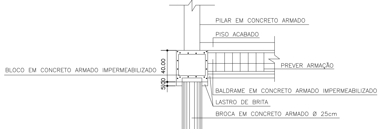
CORTE
