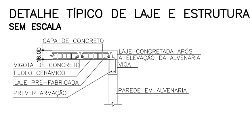
CORTE
